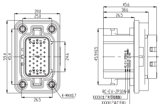
Socket RC-EV-ZP32-B-TW
