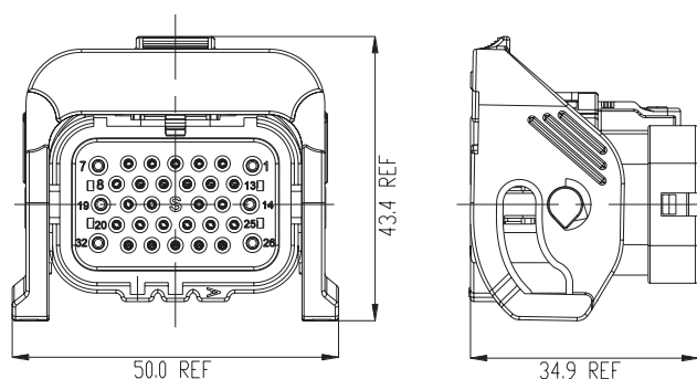
PLUG RC-EV-TS32-B-TW
