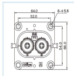
CL-HVC800-21X
