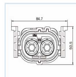
CL-HVC800-23X
