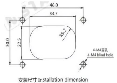
安裝尺寸 Installation dimension
